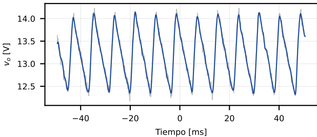
2.3.1: tab central, R_L \parallel C_2 , sobre R_L
